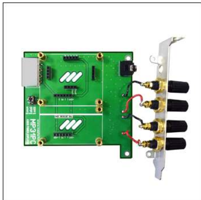
К каждой из клемм припаяйте по одному проводу с платы
