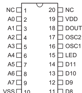
HT6014 -20 SOP-A
