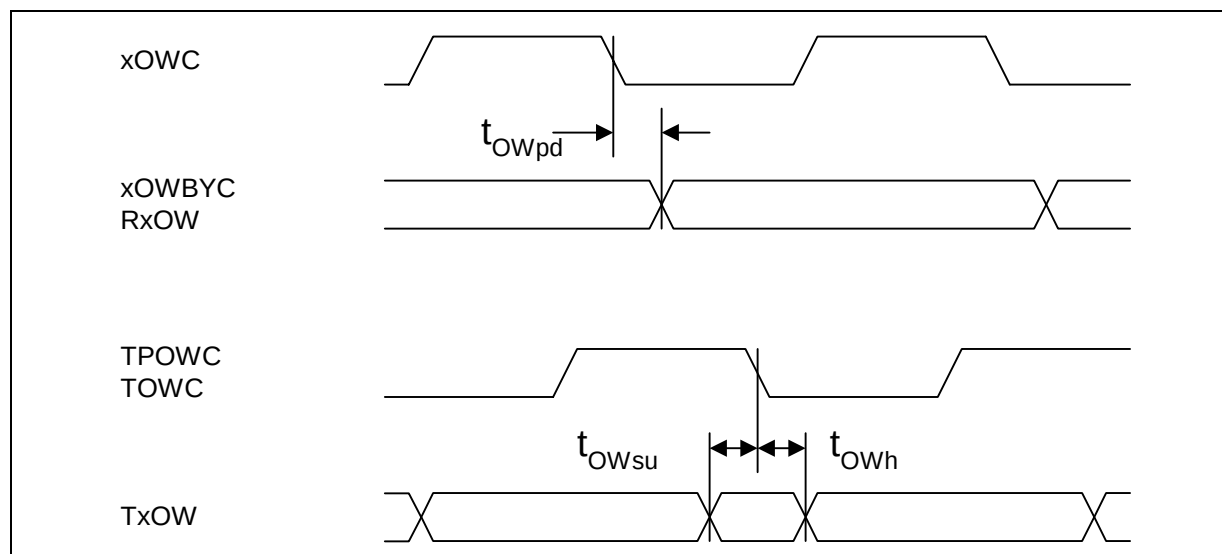
Figure 45. Orderwire E1, F1 &amp; E2, F2 &amp; F3 Timing
