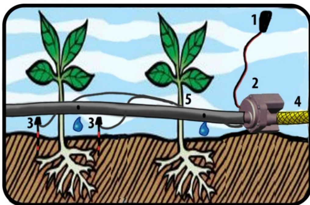
1. Источник питания; 2. Автополив «ОГО-Родник» 3. Измерительные щупы с кабелем; Система капельного полива «5» и подводящий шланг «4»
